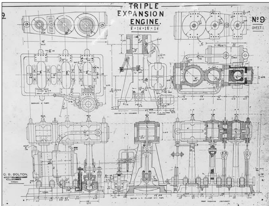
Чертеж паровой машины.
